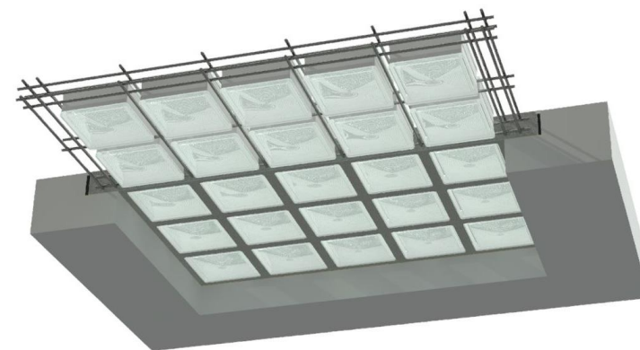
Vista inferior del panel horizontal SGB
